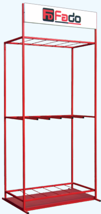
Стенд для полипропиленовой трубы Размер: 100x228x54 см. На стенде помещается 1000 м. трубы DN20x2 м.
